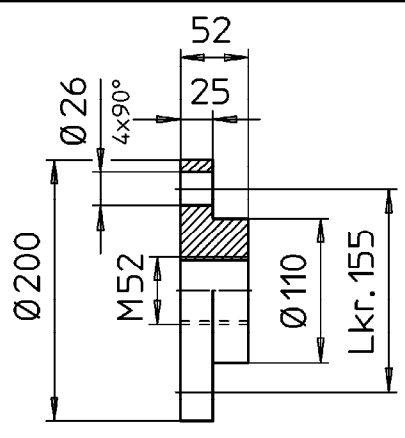
Kopfplatte
