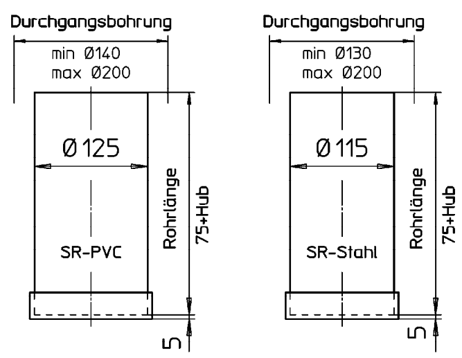
Schutzrohre
